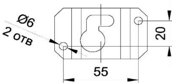
Рисунок 2.1 - Координаты отверстий крепления кронштейна модуля
