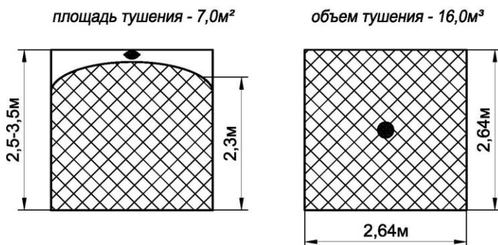
Рисунок 4 - Масштабное изображение конфигурации распыла огнетушащего порошка.
